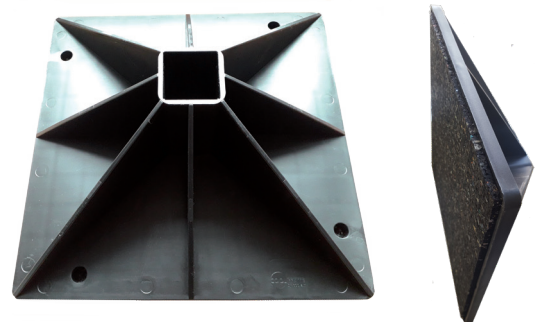
coolFRAME Fuß: Unterseite mit Anti-Vibrations-Matte
